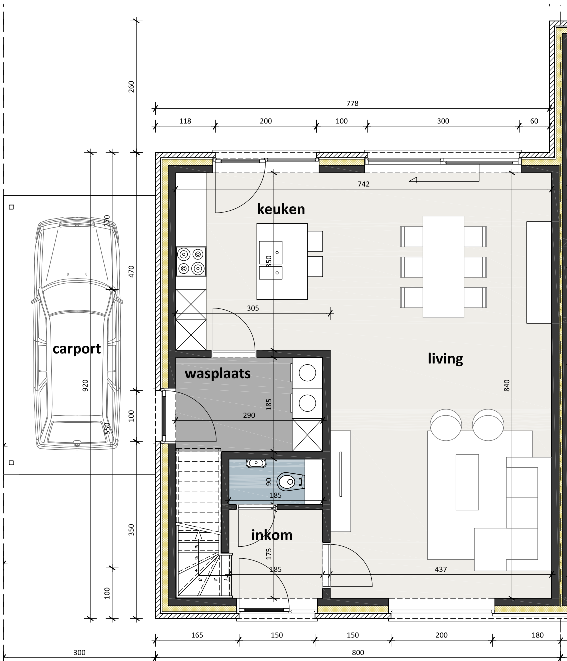
GELIJKVLOERS - LOT 9
