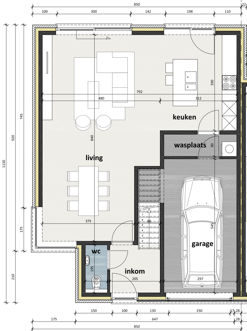
GELIJKVLOERS - LOT 7
